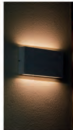
APLIQUE EXTERIOR BERN NEGRO 9712752 Luminaria de exterior para instalar en pared con luz arriba y abajo 220-240V. /12W / LED / IP54 / 580lm.
